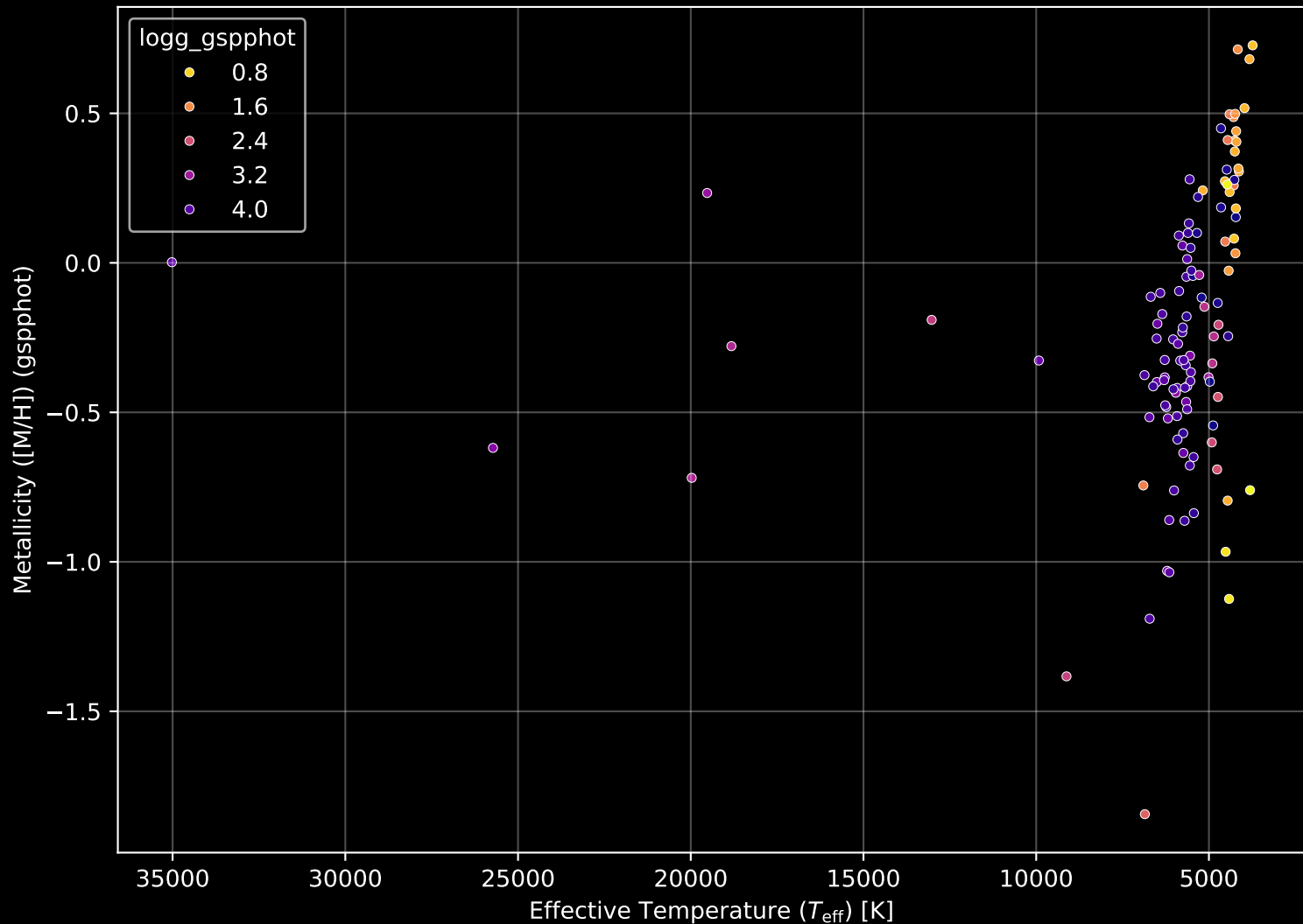
APOGEE DR17 Field: [279-32-O] Stellar Population Parameters (n= 116)
